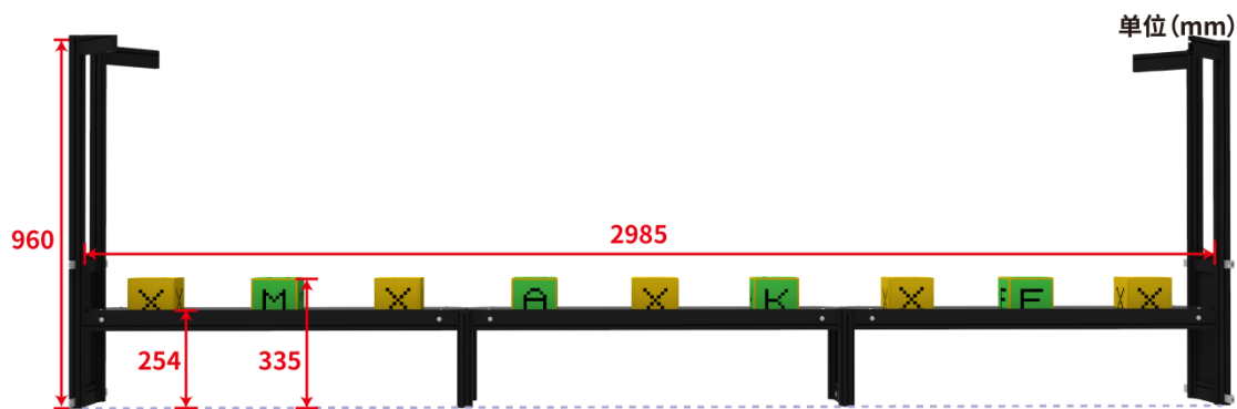
图 4.2-5 数据收集中心正视图
