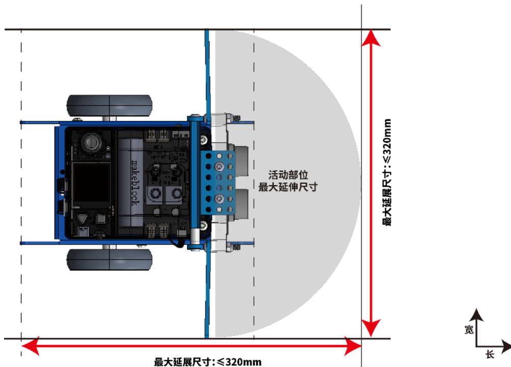
图 5.1-1 最大延伸尺寸-侧视图
